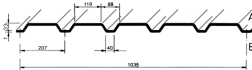
Trapezprofil 35-207 - 0,75 mm A-Seite RSL – B-Seite RAL standard - 25 µm
